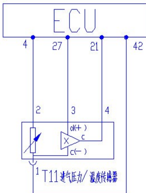
进气歧管绝对压力/进气温度传感器
