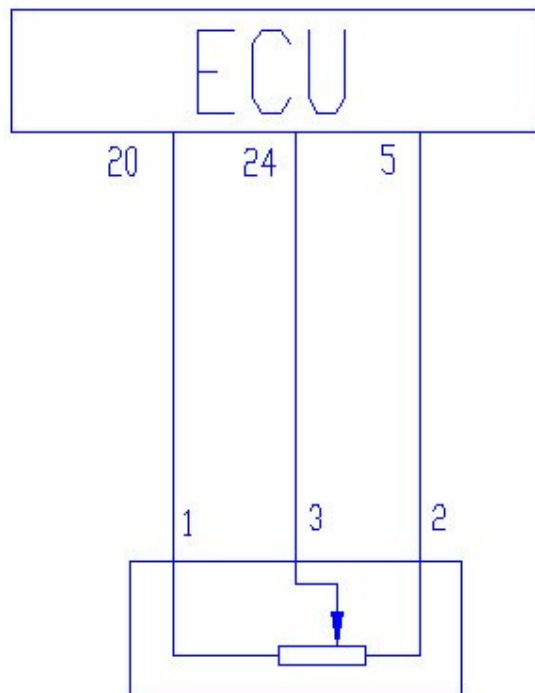
T11 节气门位置传感器
