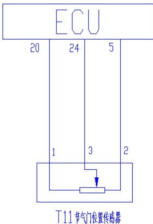
节气门位置传感器电路图
