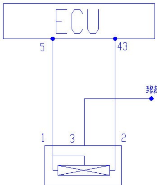
T11 水温传感器
