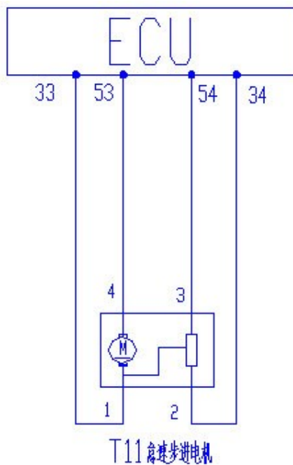
怠速执行器步进电机电路图
