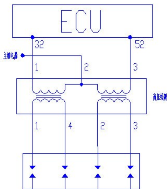
T11 点火线圈组
