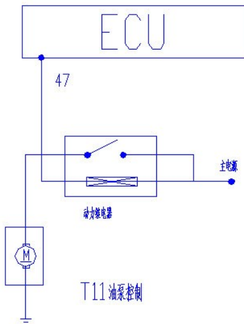
电动燃油泵图
