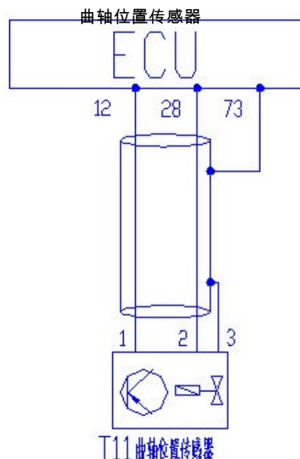
曲轴位置传感器电路图
